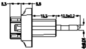
EU Plug
